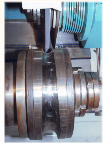
Die Groove Grinding Machine
